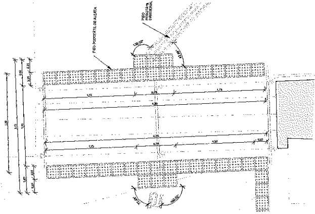
3 | PLANTA DE ACESSIBILIDADE DETALHE 2 1:1,25
